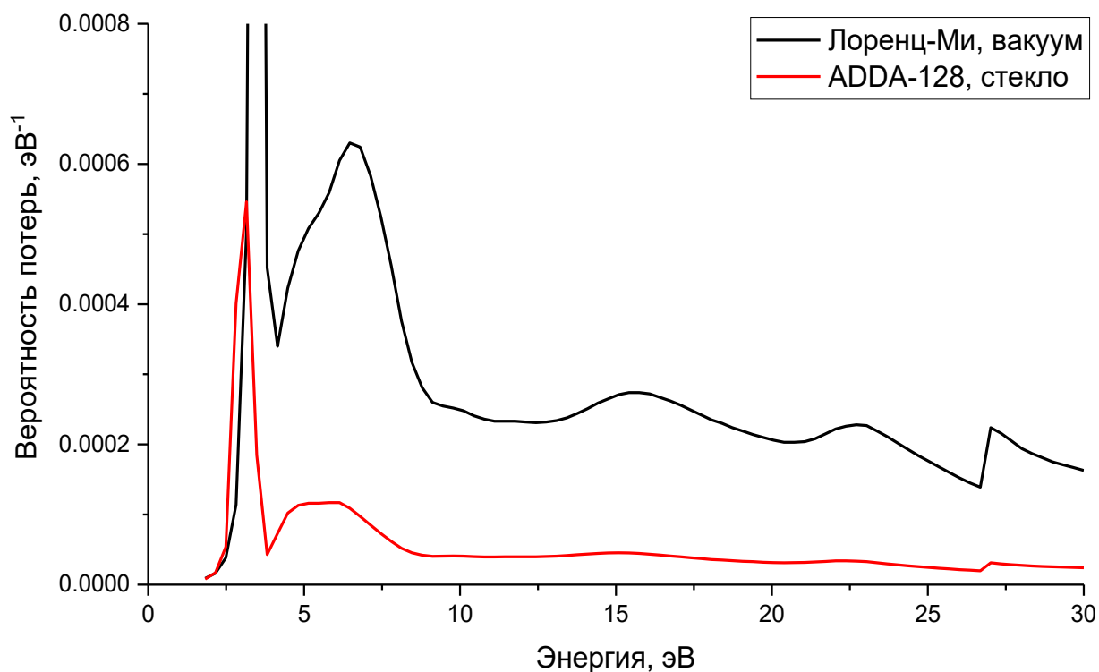
Рис. 7. Спектры EELS, полученные точным решением по теории Лоренца-Ми в вакууме и моделированием в ADDA в стекле с коэффициентом преломления n = 1.5 . Электрон с энергией 100 кэВ пролетает в 6 нм от центра шара из серебра с радиусом 5 нм.
